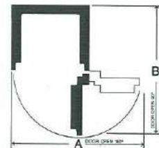
Door Swing Diagram
